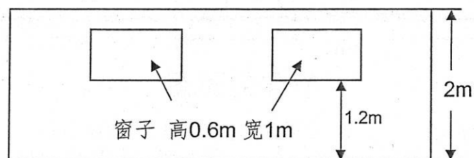
牛舍后墙示意图
