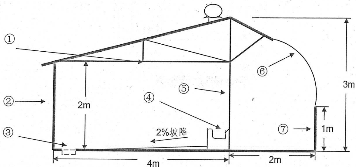
牛舍剖面图
