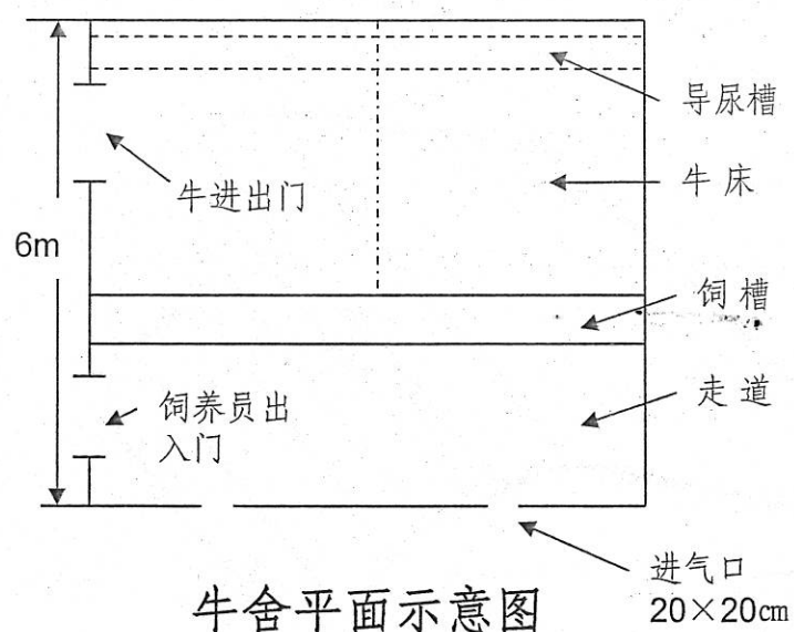
单列式暖棚牛舍示意图 (2-2)
